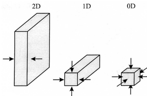
Рис.3. Пространственное ограничение волновых функций в двумерных (2D), одномерных (1D) и нуль-мерных (0D) системах.
